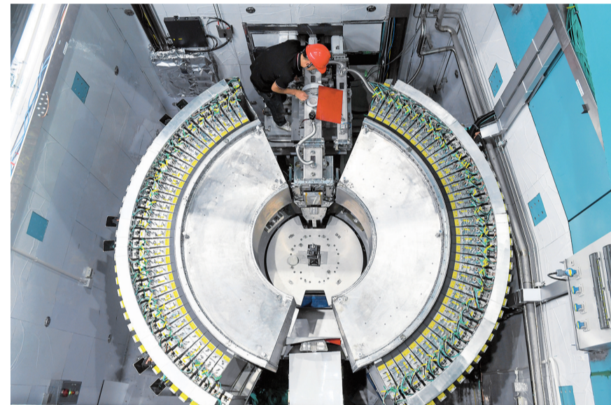
7月8日,工作人员为高压中子衍射仪中子导管包裹柔性碳化硼,吸收杂散中子。近日,国家重大科技基础设施——中国散裂中子源高分辨中子衍射仪、高压中子衍射仪成功出束。这两台谱仪设备的研制、安装成功,将显著增强中国散裂中子源的多学科研究能力。【新华社记者 毛思倩 摄】
